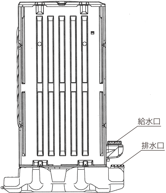
B 立面図
