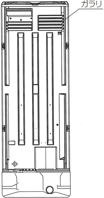
C 正面図
