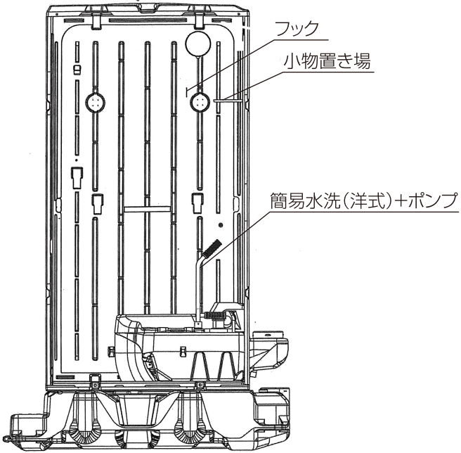
A-C 断面図
