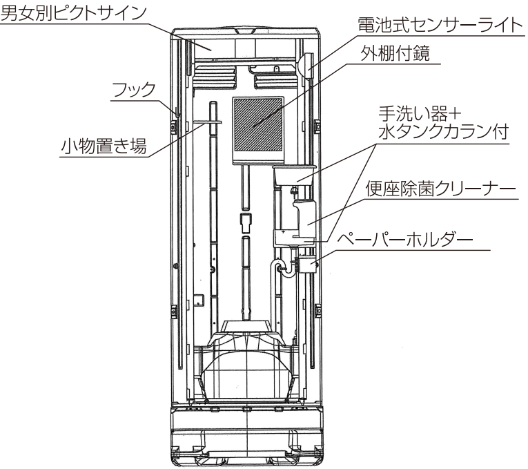
D-B 断面図
