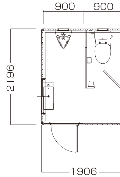
平面図
