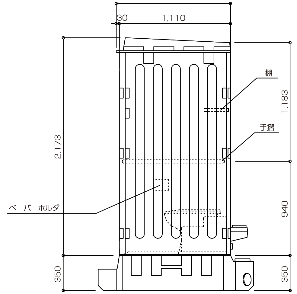
側面図
