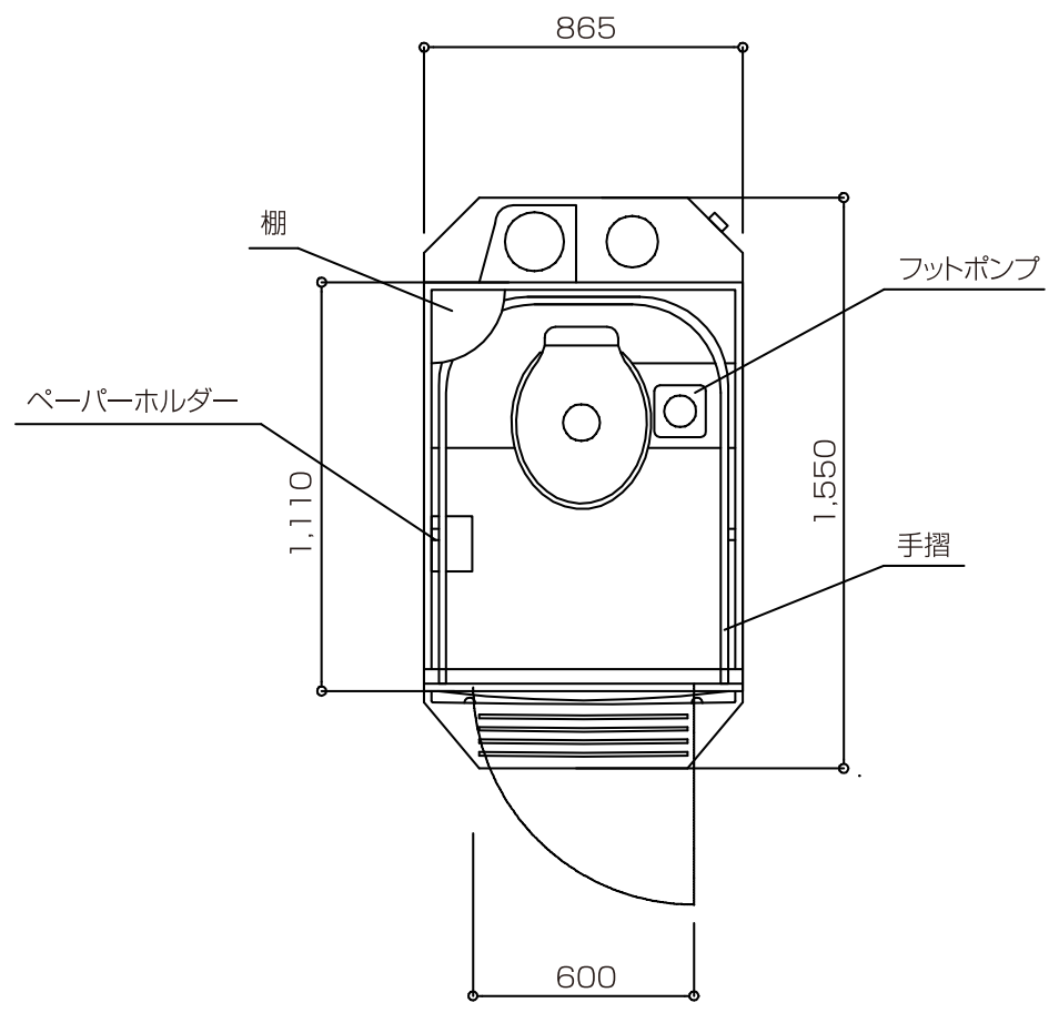
平面図
