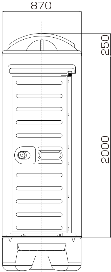
正面図
