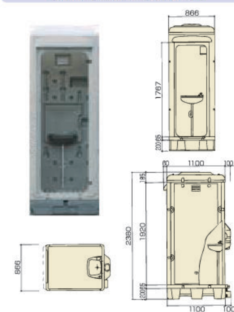
水洗式手洗い室(WOF-手)
