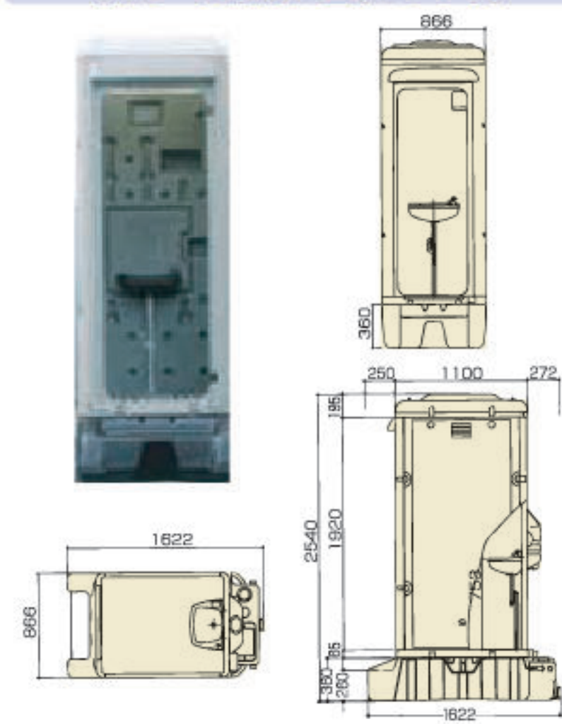
水洗式手洗い室(WOF-手)
