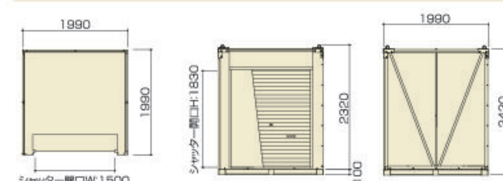
PS-2型 L1990×W1990×H2420
