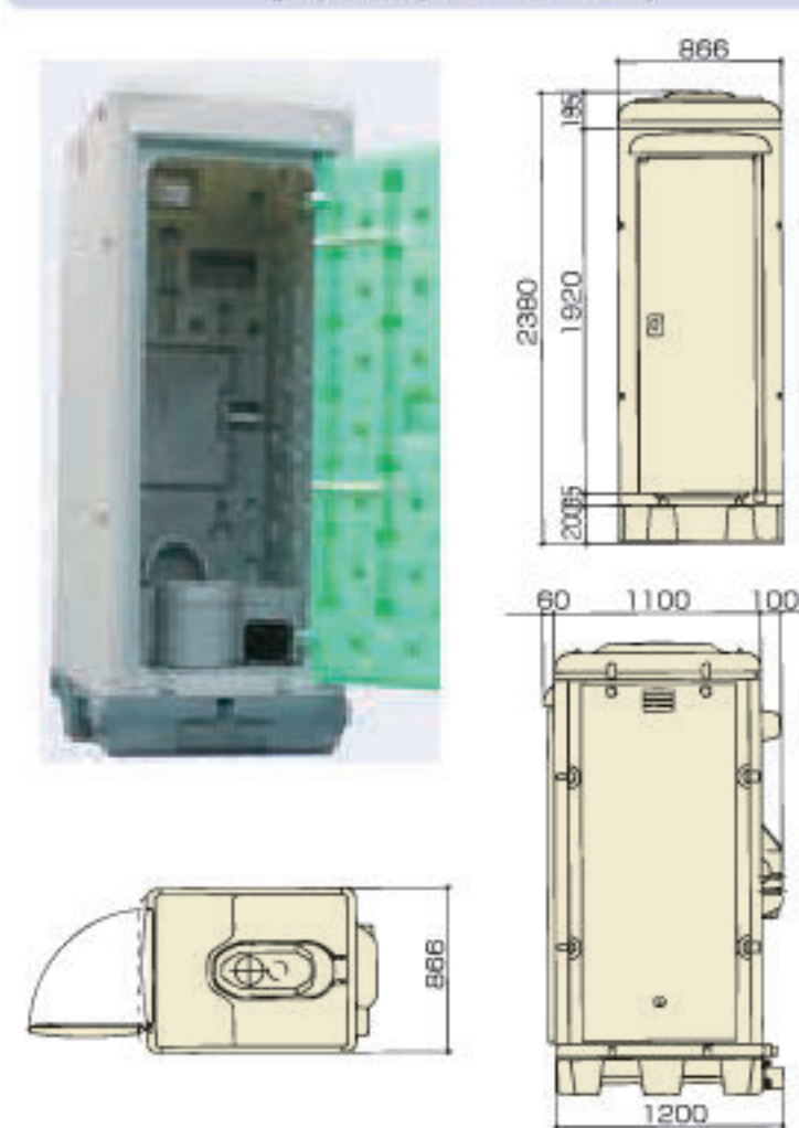
水洗式(WOF-1型)
