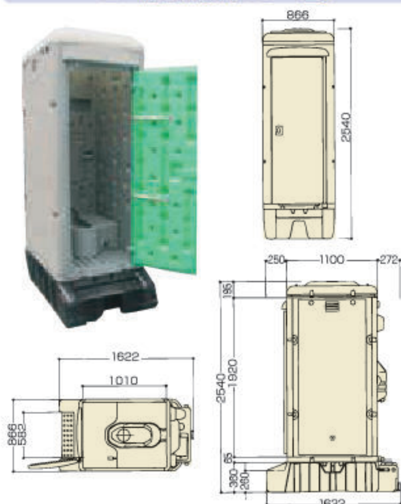
水洗式(WOF-1型)
