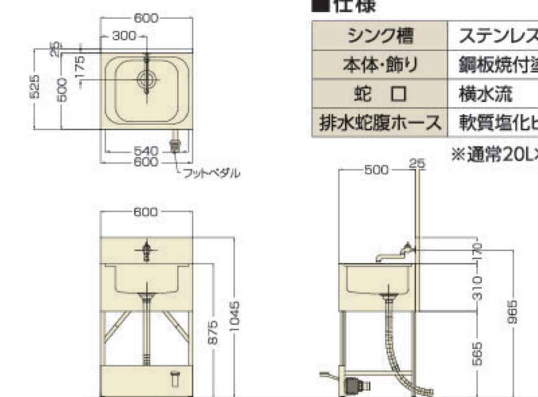
フットポンプ式シンク HC-1(F)型 W600×D525×H1045
