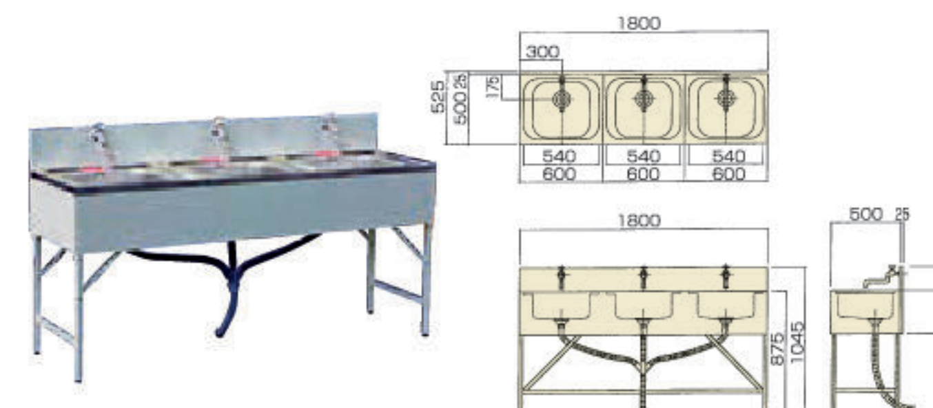
三槽シンク(HC-3型) W1800×D525×H1045
