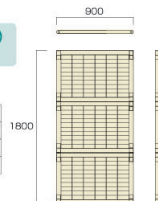
※(例) L字型3枚取付の時
