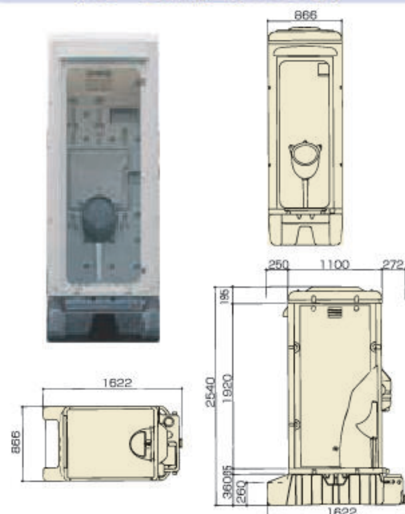
水洗式小便室(WOF-小)
