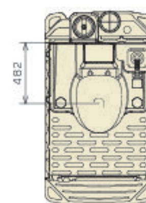
簡易水洗 洋式
