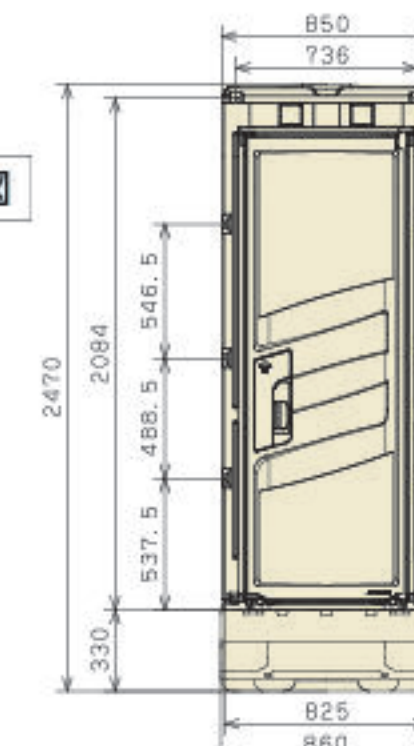
簡易水洗 正面図
