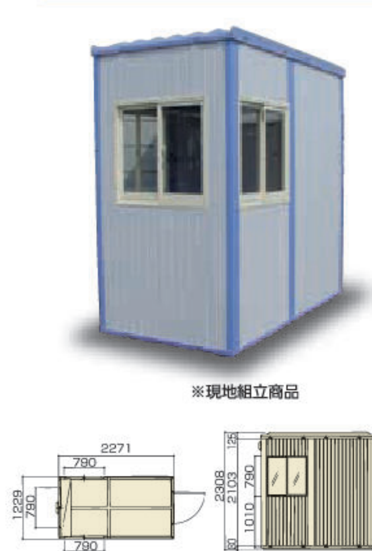
LGB型 W2271×D1229×H2308
