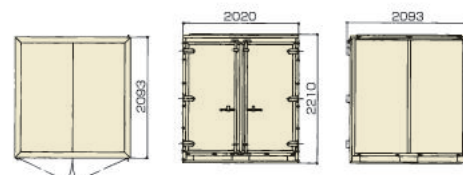
KC-20型 W2020×D2093×H2210
