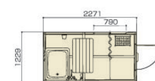
LBA型 W1229×D2271×H2308
