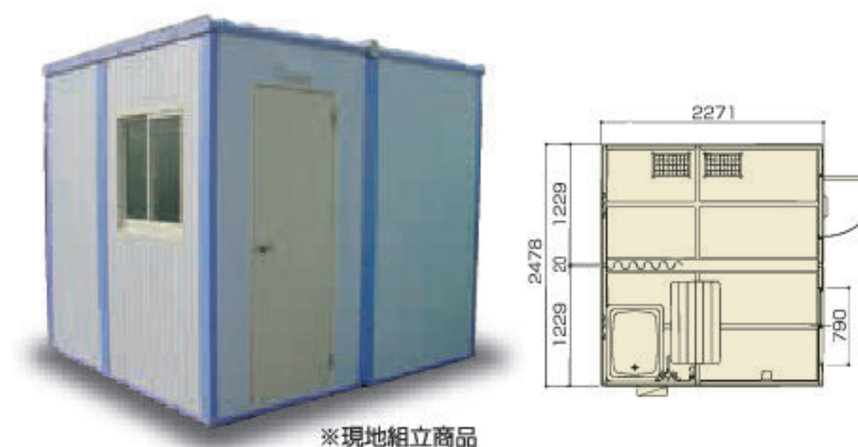
LBB型 W2478×D2271×H2308
