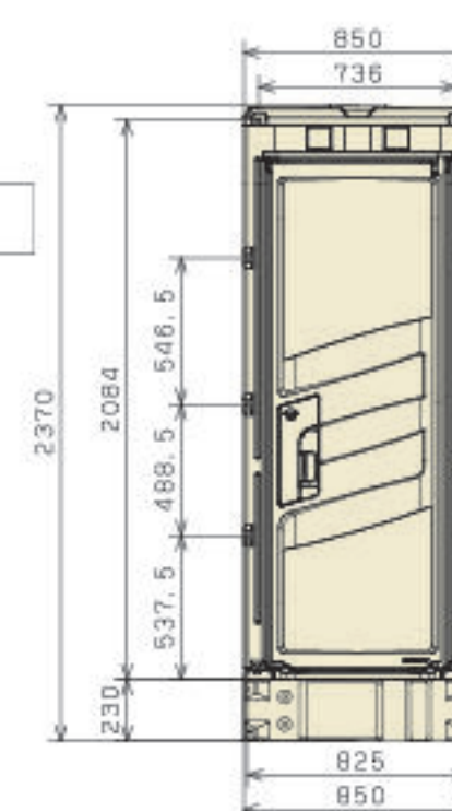
本水洗 正面図
