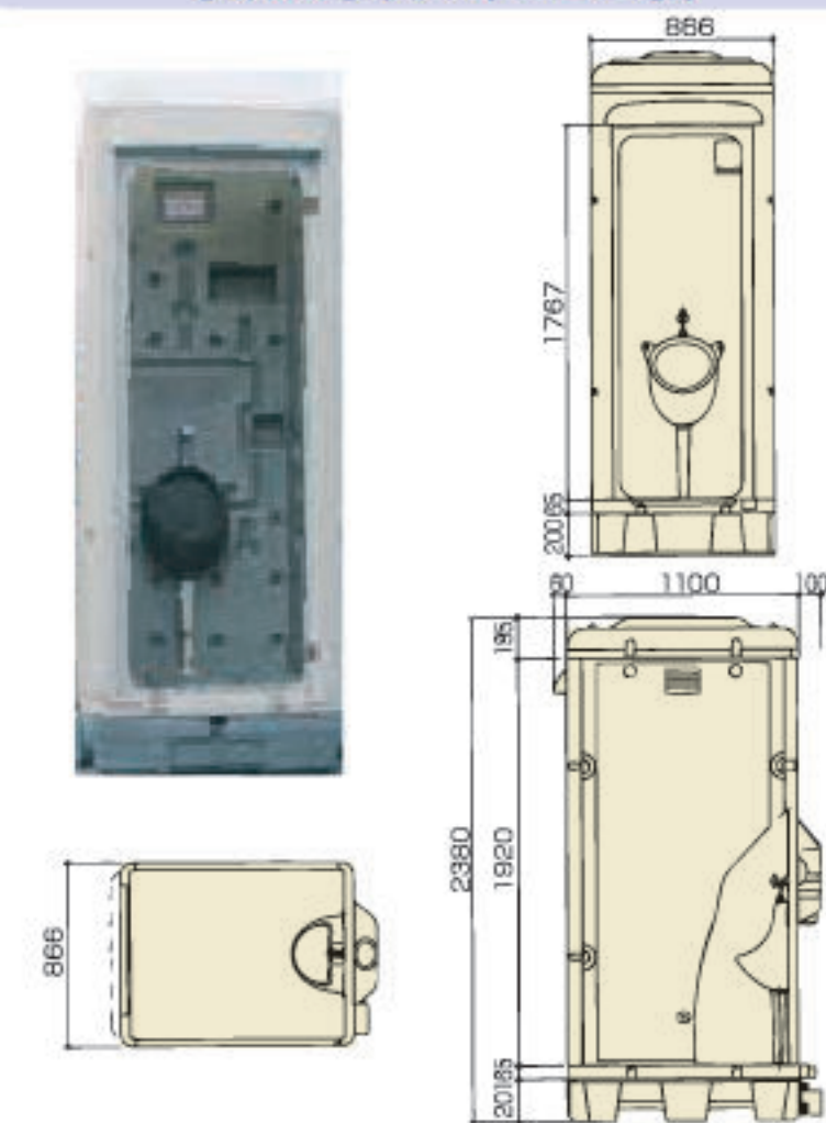
水洗式小便室(WOF-小)
